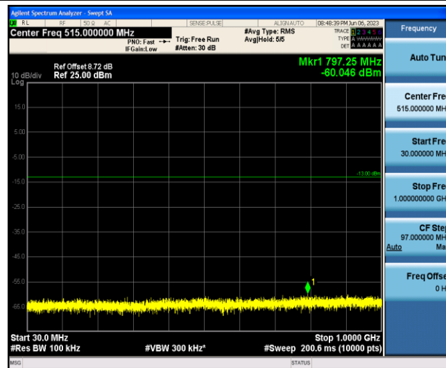
Band2-20MHz-QPSK-18700-1-0-Low-30-1000--60.05-PASS
