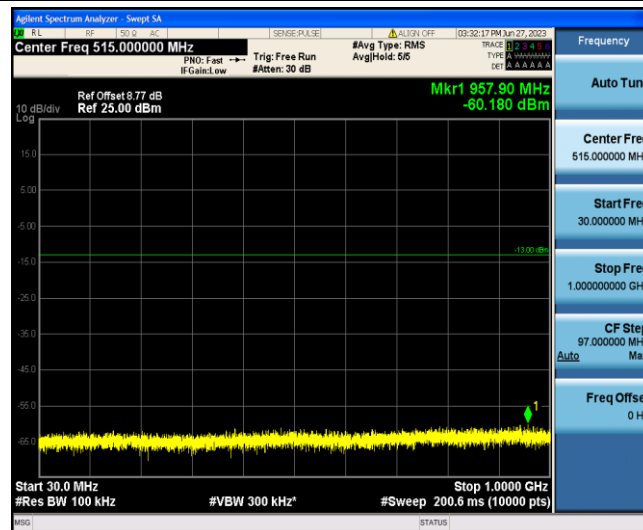
Band4-1.4MHz-QPSK-19957-1-0-Low-30-1000--60.18-PASS
