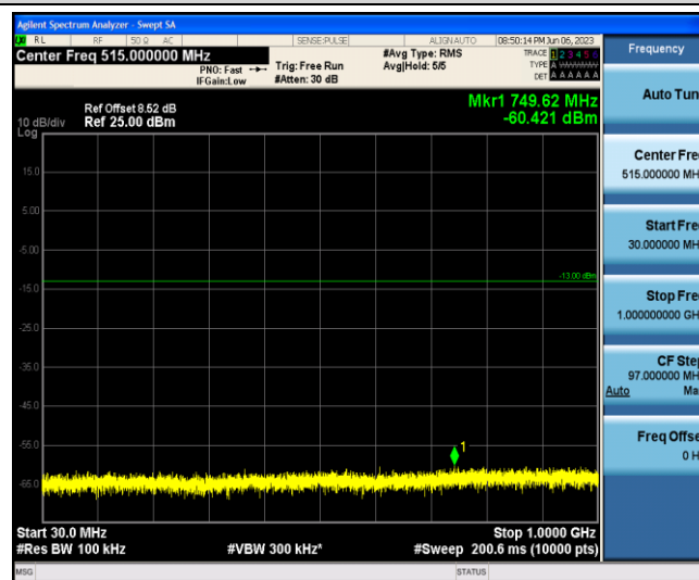
Band2-20MHz-QPSK-19100-1-0-Low-30-1000--60.42-PASS
