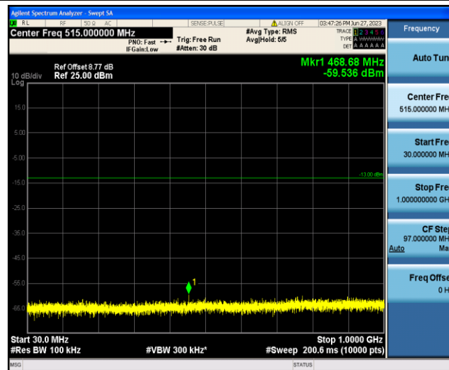
Band4-3MHz-QPSK-19965-1-0-Low-30-1000--59.54-PASS
