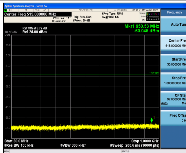
Band2-20MHz-16QAM-18900-1-0-Low-30-1000--60.05-PASS
