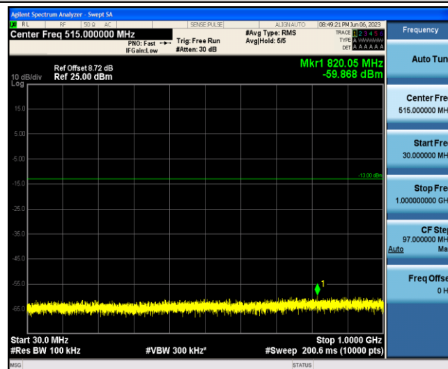
Band2-20MHz-QPSK-18900-1-0-Low-30-1000--59.87-PASS
