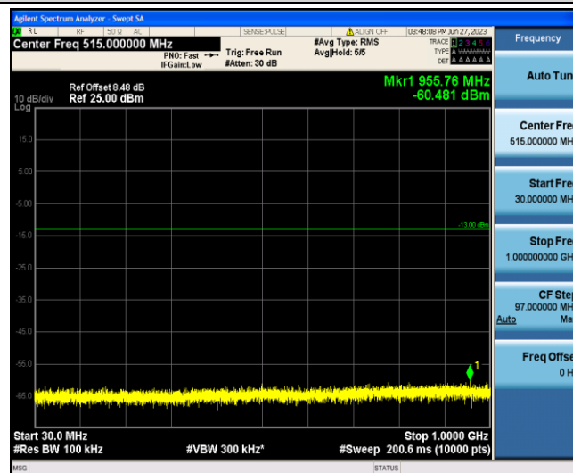
Band4-3MHz-QPSK-20175-1-0-Low-30-1000--60.48-PASS
