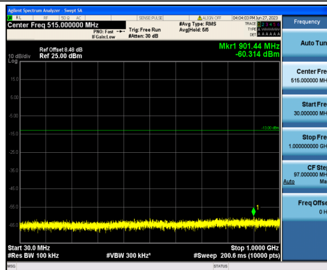
Band4-5MHz-QPSK-20375-1-0-Low-30-1000--60.31-PASS
