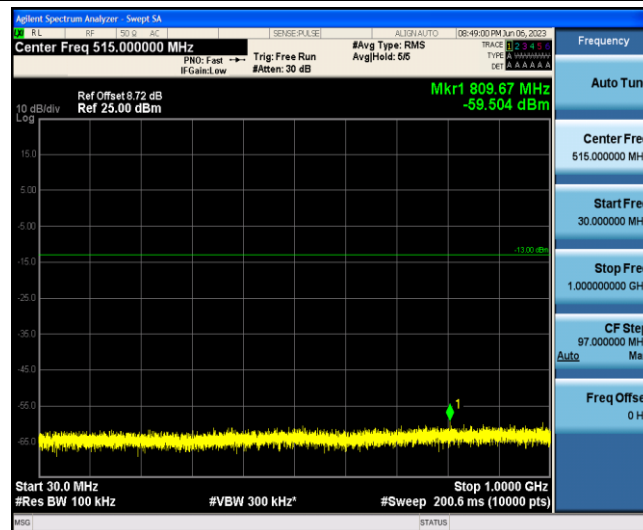
Band2-20MHz-16QAM-18700-1-0-Low-30-1000--59.5-PASS
