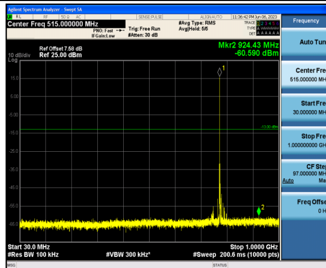
Band13-10MHz-16QAM-23230-1-0-Low-30-1000--60.59-PASS
