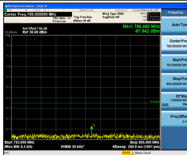
Band13-5MHz-16QAM-23230-1-0-Low-793-805--61.64-PASS
