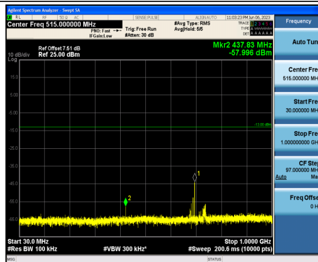
Band12-10MHz-QPSK-23130-1-0-Low-30-1000--58-PASS
