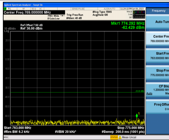
Band13-5MHz-QPSK-23230-1-0-Low-763-775--62.43-PASS
