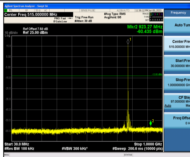
Band13-10MHz-QPSK-23230-1-0-Low-30-1000--60.44-PASS
