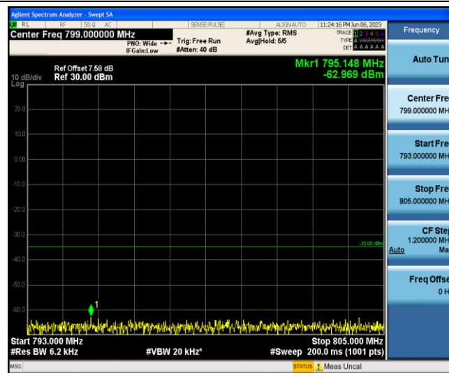
Band13-5MHz-QPSK-23230-1-0-Low-793-805--62.97-PASS
