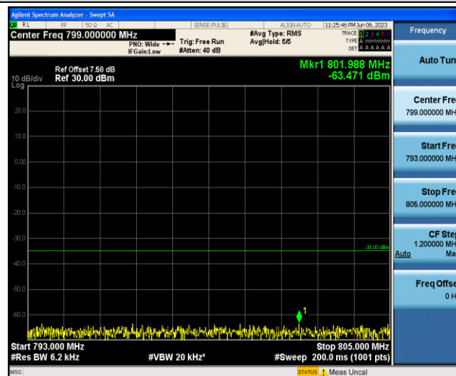
Band13-5MHz-16QAM-23255-1-0-Low-793-805--63.47-PASS
