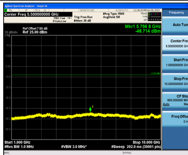
Band13-10MHz-QPSK-23230-1-0-Low-1000-10000--48.71-PASS
