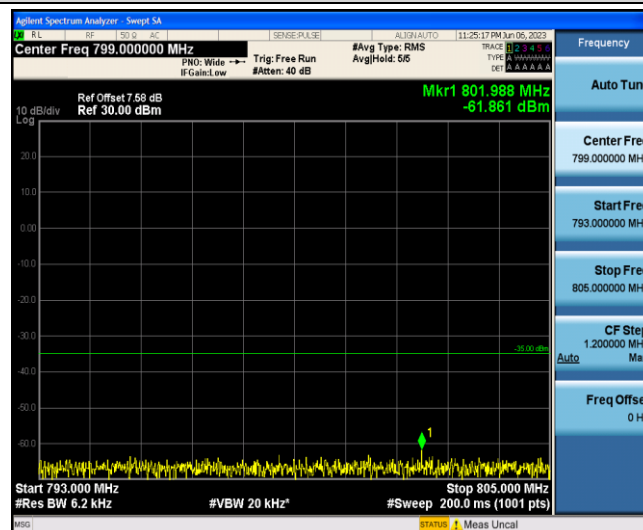
Band13-5MHz-QPSK-23255-1-0-Low-793-805--61.86-PASS
