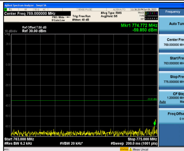
Band13-10MHz-QPSK-23230-1-0-Low-763-775--59.85-PASS
