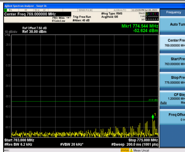
Band13-5MHz-QPSK-23205-1-0-Low-763-775--52.62-PASS
