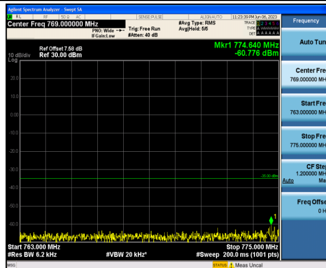
Band13-5MHz-16QAM-23205-1-0-Low-763-775--60.78-PASS
