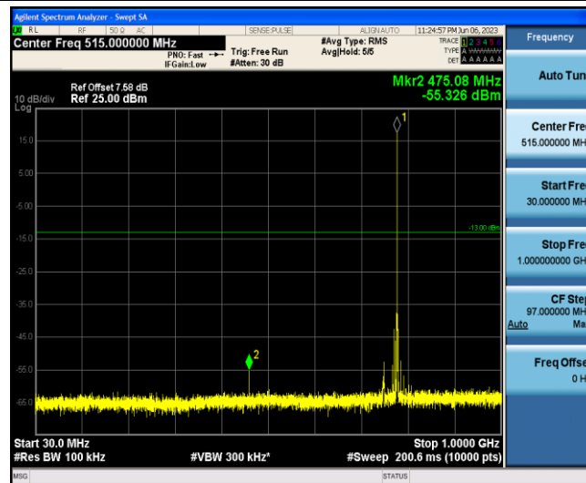
Band13-5MHz-QPSK-23255-1-0-Low-30-1000--55.33-PASS
