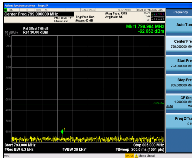
Band13-5MHz-QPSK-23205-1-0-Low-793-805--62.65-PASS
