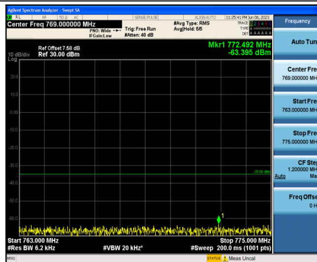
Band13-5MHz-16QAM-23255-1-0-Low-763-775--63.4-PASS
