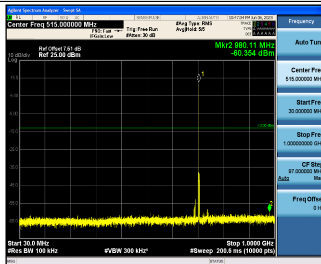
Band12-5MHz-QPSK-23155-1-0-Low-30-1000--60.35-PASS
