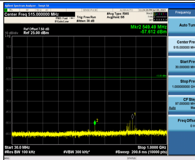
Band13-5MHz-16QAM-23230-1-0-Low-30-1000--57.61-PASS
