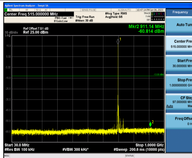
Band12-5MHz-16QAM-23095-1-0-Low-30-1000--60.81-PASS
