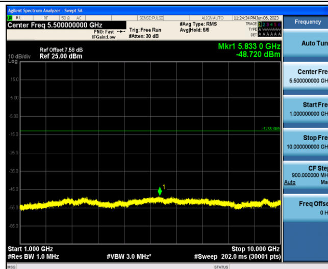
Band13-5MHz-16QAM-23230-1-0-Low-1000-10000--48.72-PASS
