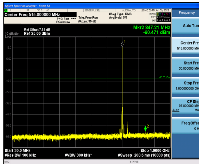
Band12-5MHz-QPSK-23095-1-0-Low-30-1000--60.47-PASS
