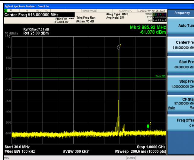
Band12-10MHz-QPSK-23060-1-0-Low-30-1000--61.08-PASS
