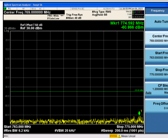
Band13-10MHz-16QAM-23230-1-0-Low-763-775--60.87-PASS
