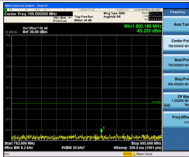
Band13-5MHz-16QAM-23205-1-0-Low-793-805--63.23-PASS
