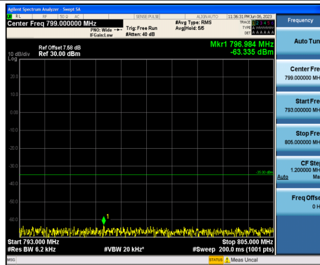
Band13-10MHz-QPSK-23230-1-0-Low-793-805--63.34-PASS
