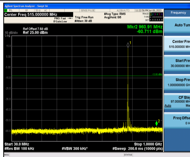
Band13-5MHz-QPSK-23205-1-0-Low-30-1000--60.71-PASS
