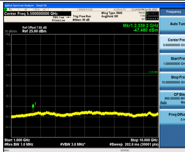
Band13-5MHz-QPSK-23230-1-0-Low-1000-10000--47.48-PASS
