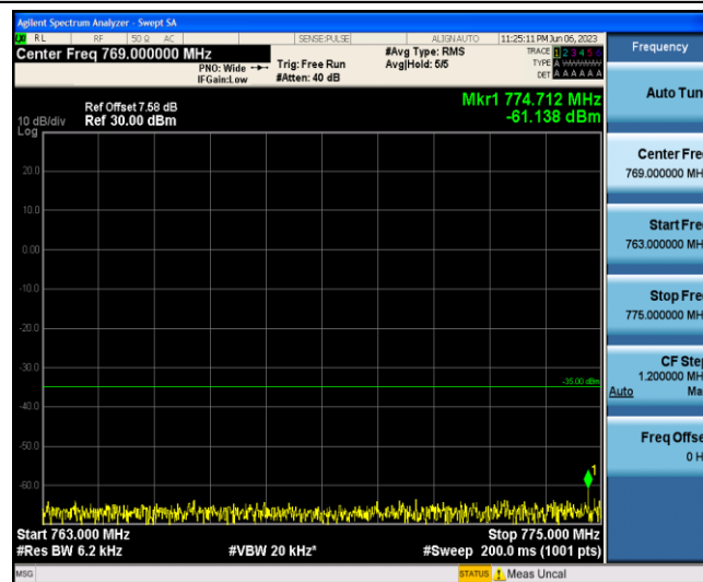
Band13-5MHz-QPSK-23255-1-0-Low-763-775--61.14-PASS
