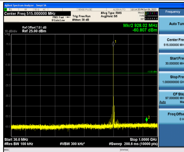
Band12-1.4MHz-QPSK-23095-1-0-Low-30-1000--60.81-PASS
