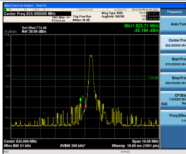
Band5-3MHz-16QAM-20415-1-0-Low--35.18-PASS
