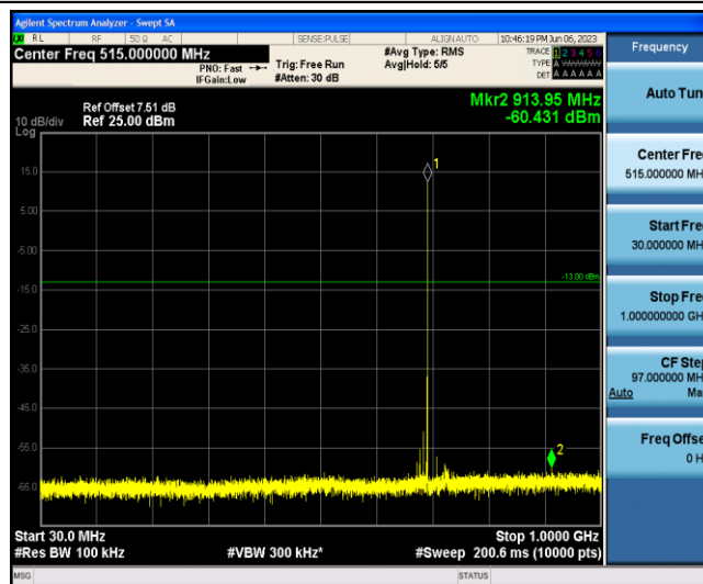
Band12-5MHz-QPSK-23035-1-0-Low-30-1000--60.43-PASS
