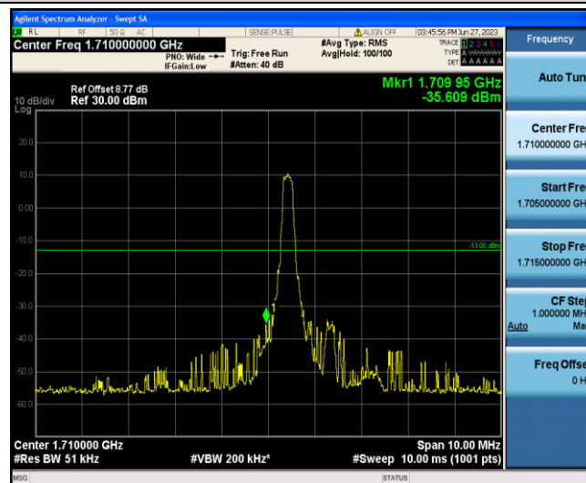
Band4-3MHz-QPSK-19965-1-0-Low--35.61-PASS
