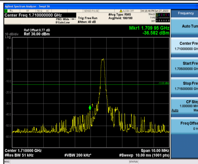
Band4-10MHz-16QAM-20000-1-0-Low--36.58-PASS
