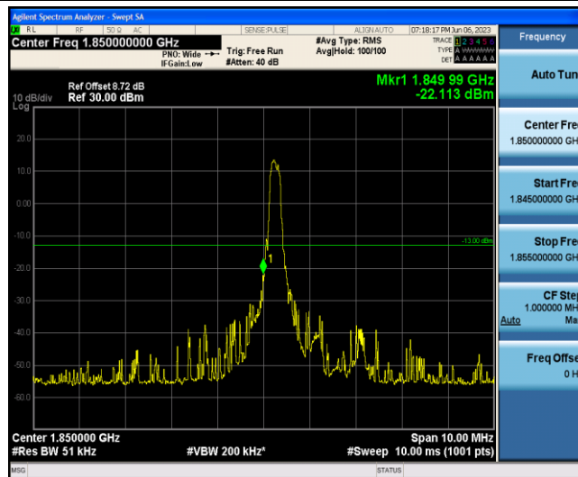
Band2-1.4MHz-QPSK-18607-1-0-Low--22.11-PASS
