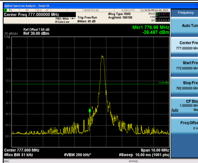
Band13-10MHz-16QAM-23230-1-0-Low--39.49-PASS
