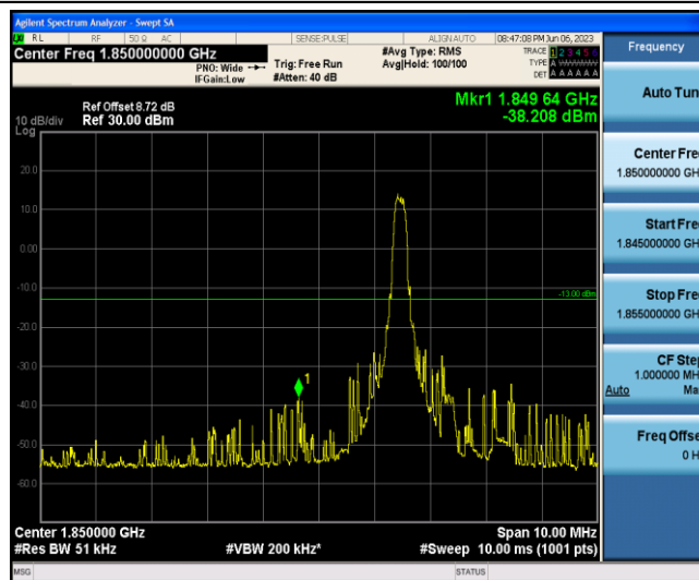
Band2-20MHz-QPSK-18700-1-0-Low--38.21-PASS
