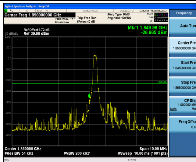
Band2-5MHz-QPSK-18625-1-0-Low--26.87-PASS
