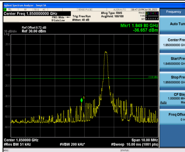
Band2-20MHz-16QAM-18700-1-0-Low--36.66-PASS
