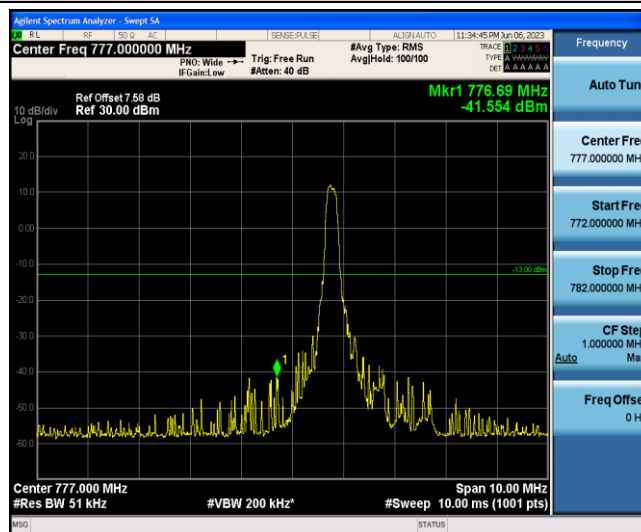
Band13-10MHz-QPSK-23230-1-0-Low--41.55-PASS
