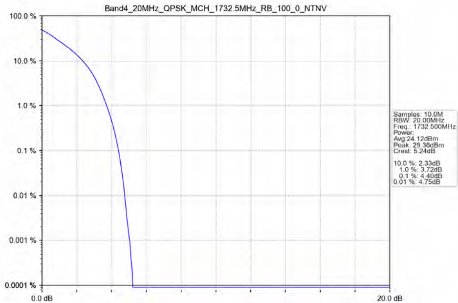
Band4_20MHz_QPSK_MCH_1732.5MHz_RB_100_0_NTNV
