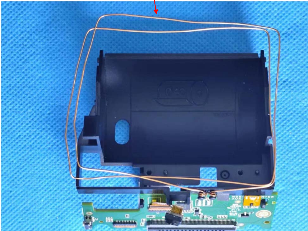
NFC Antenna
