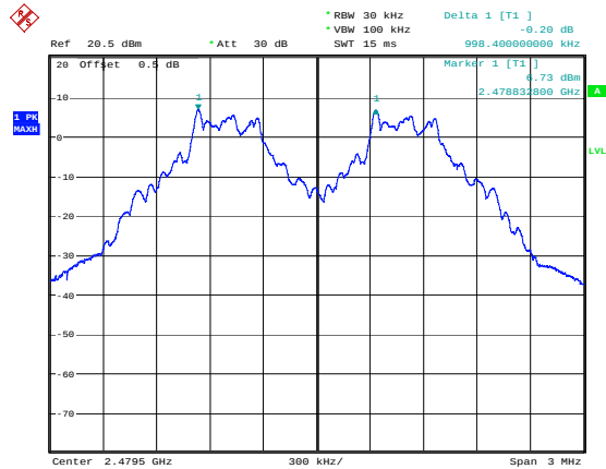
GFSK_High 0.998MHz
