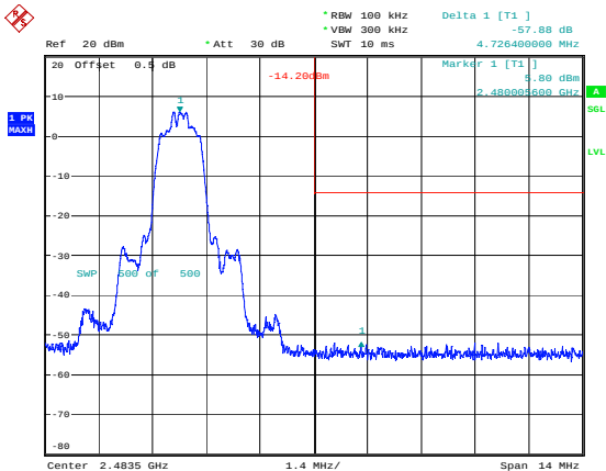
\pi/4 -DQPSK_High 57.88dB
