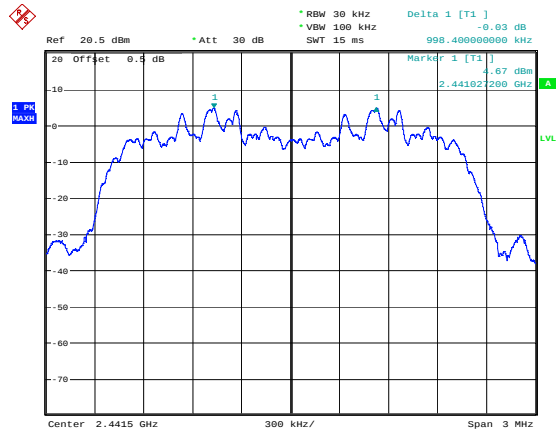
\pi/4 -DQPSK_Middle 0.998MHz
