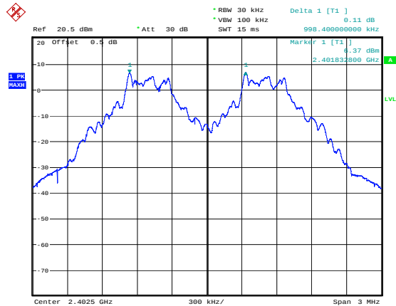
GFSK_Low 0.998MHz
