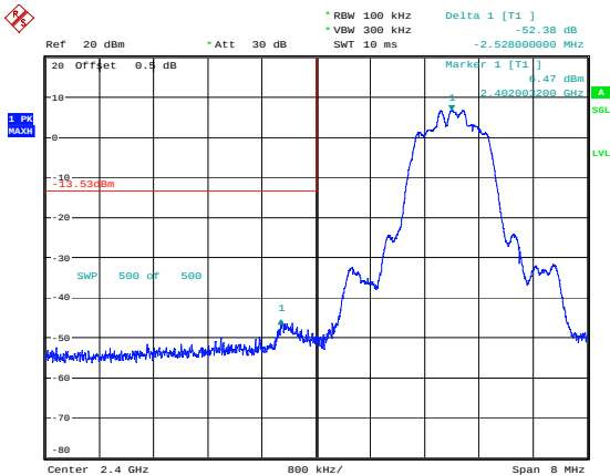
\pi/4 -DQPSK_Low 52.38dB
