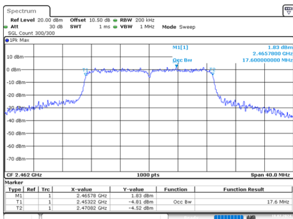
n20_2462MHz_Chain 0 17.600MHz
