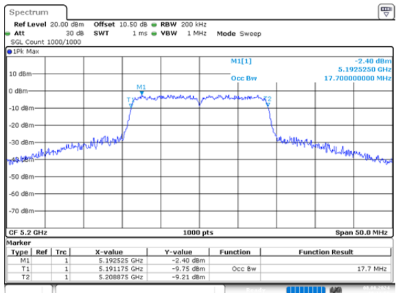
n20_5200MHz_Chain 0 17.700MHz
