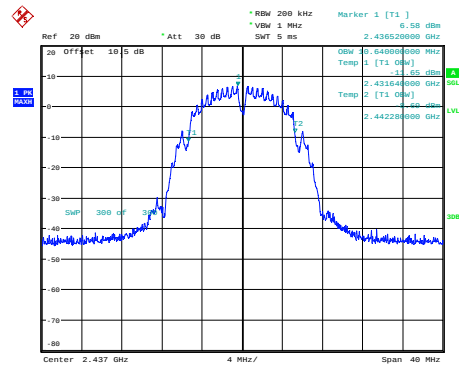
b_2437MHz_Chain 0
