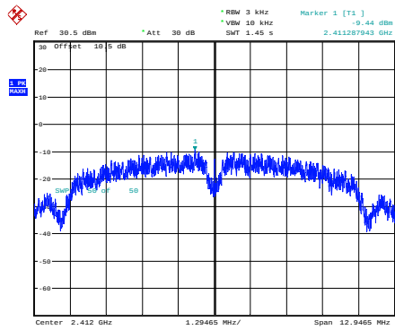
b_2412MHz_Chain 0
