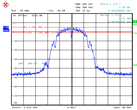
b_2412MHz_Chain 0
