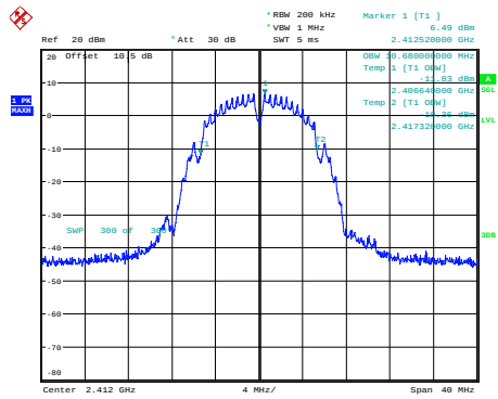
b_2412MHz_Chain 0
