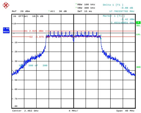
n20_2462MHz_Chain 0
