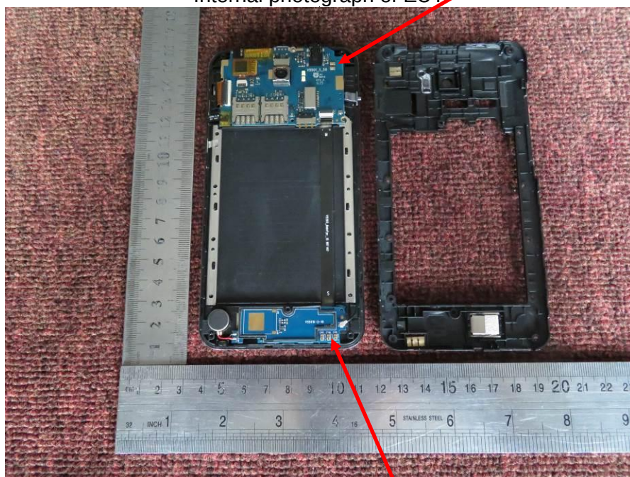
GSM/WCDMA Antenna
