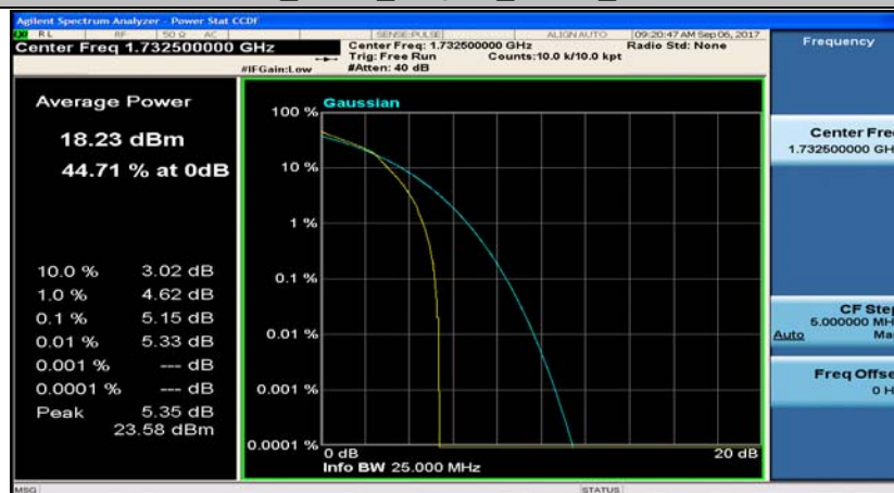
Band4_10MHz_QPSK_20175_1RB#0
