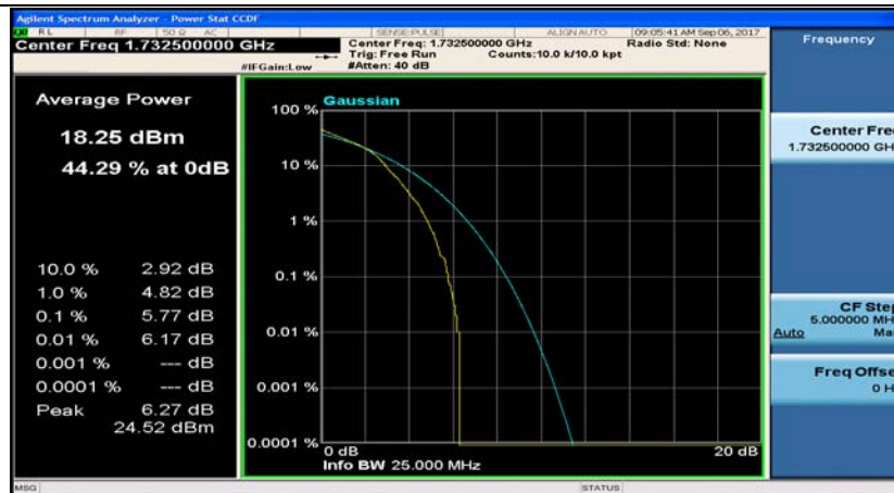
Band4_20MHz_QPSK_20175_1RB#0
