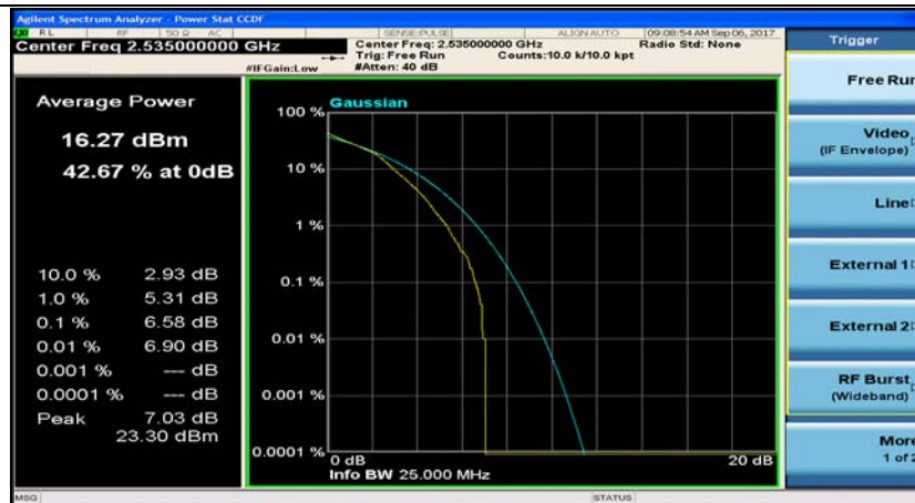
Band7_20MHz_QPSK_21100_100RB#0
