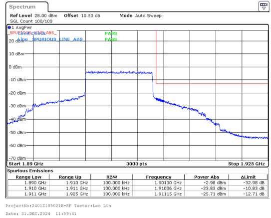
Band 2 10MHz/1905.0/High QPSK 50@0
