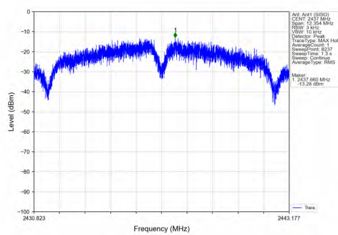
802.11b_MCH_2437MHz_Ant1 (SISO)_NTNV
