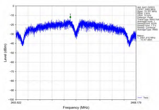
802.11b_HCH_2462MHz_Ant1 (SISO)_NTNV
