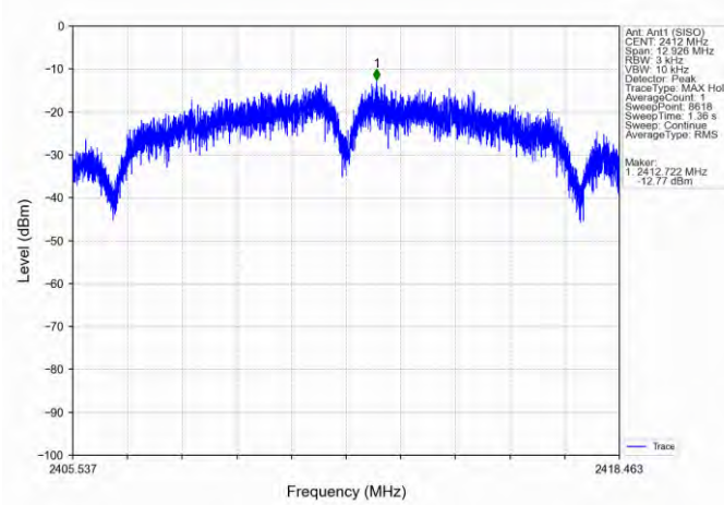
802.11b_LCH_2412MHz_Ant1 (SISO)_NTNV
