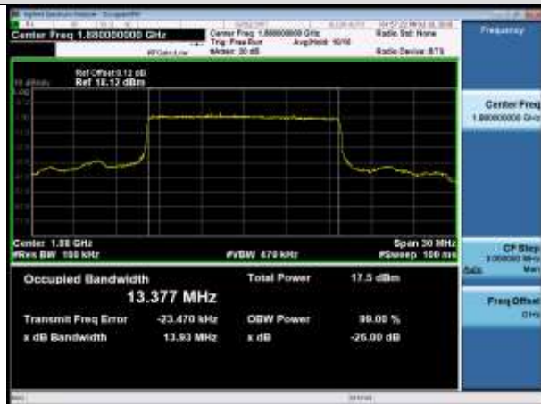
MCH_QPSK_75RB#0
