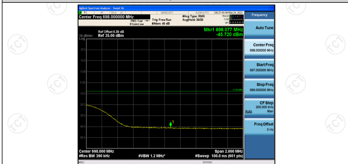
Band71-20MHz-QPSK-133372-1RB#99
