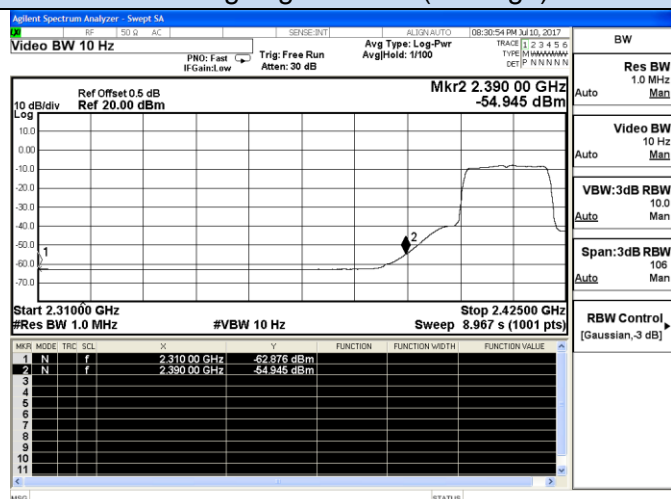
802.11n-HT20-Low channel(Average)
