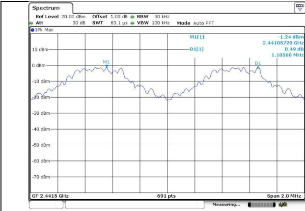
GFSK
