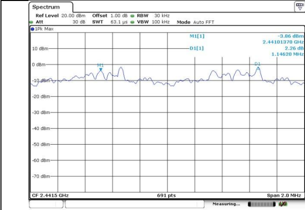
8DPSK
