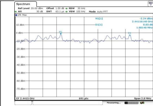
\pi/4 DQPSK
