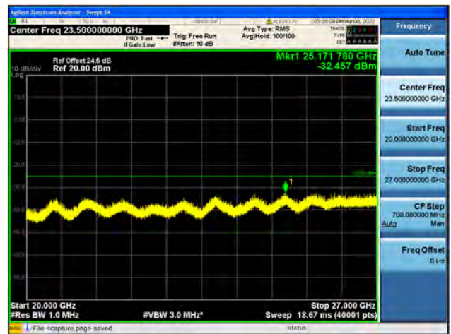
Band41-20G-27G / 20MHz / Low CH / 64QAM
