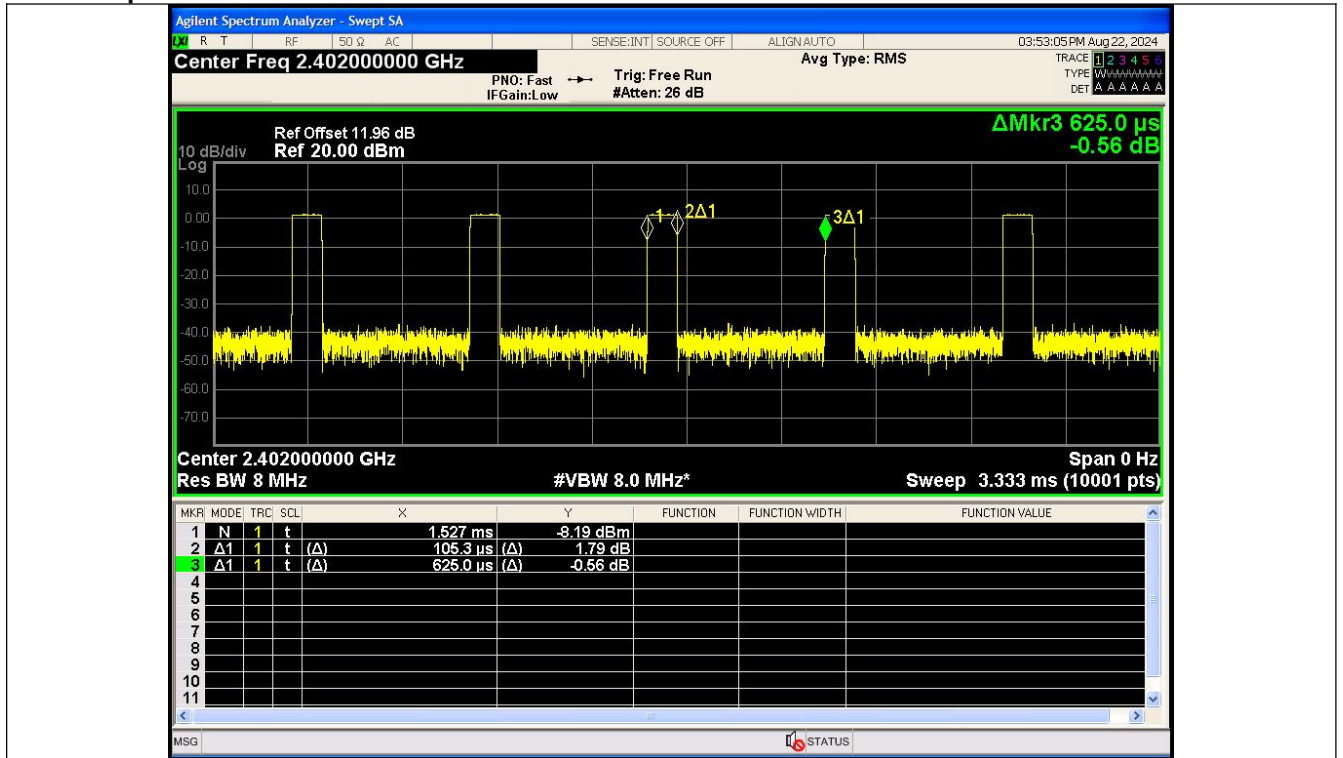
BLE 1M_Channel 0
