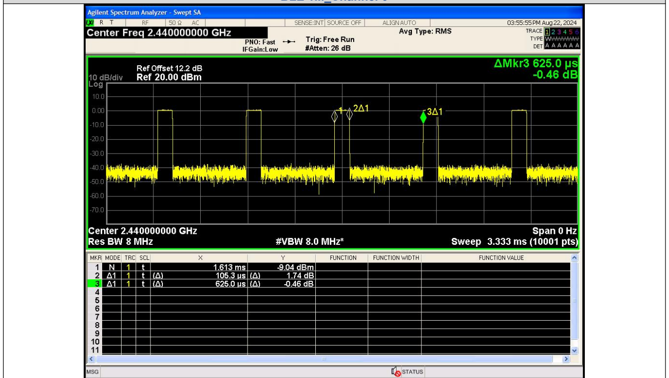
BLE 1M_Channel 19
