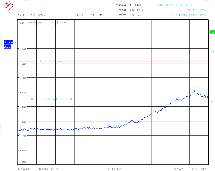
Band2 GSM UL Left Side Pre AGC
