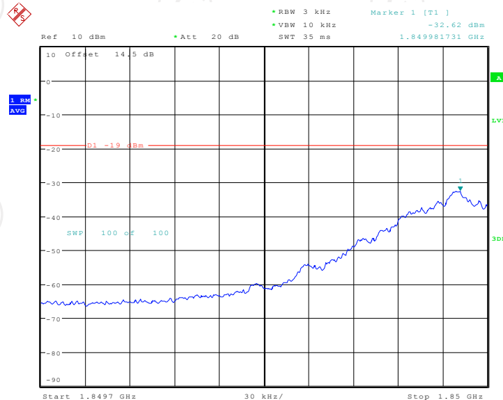
Band2 GSM UL Left Side Max. Input
