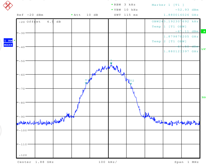
Band2 GSM UL Input
