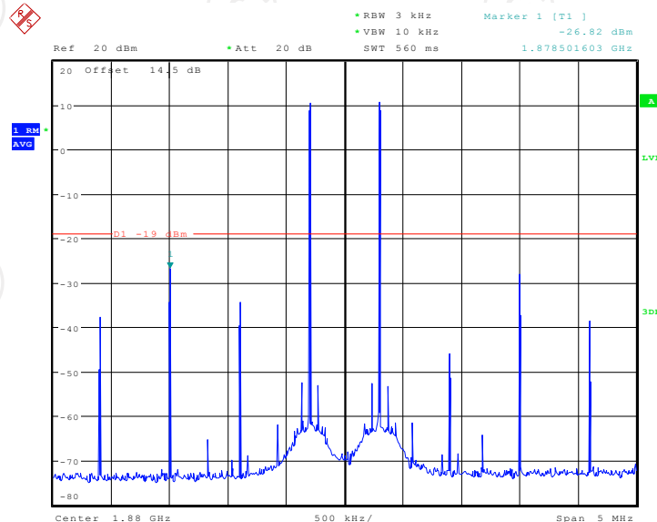
Band2 AGC +10dB, UL
