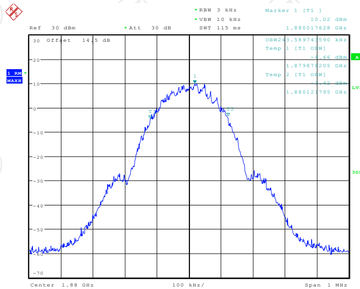
Band2 GSM UL output
