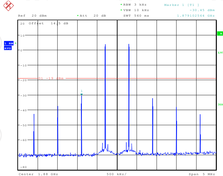
Band2 Pre AGC, UL
