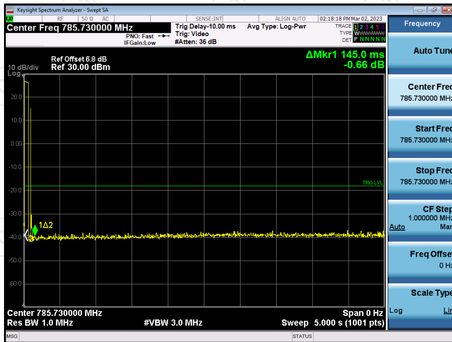
Upper700MHz UL
