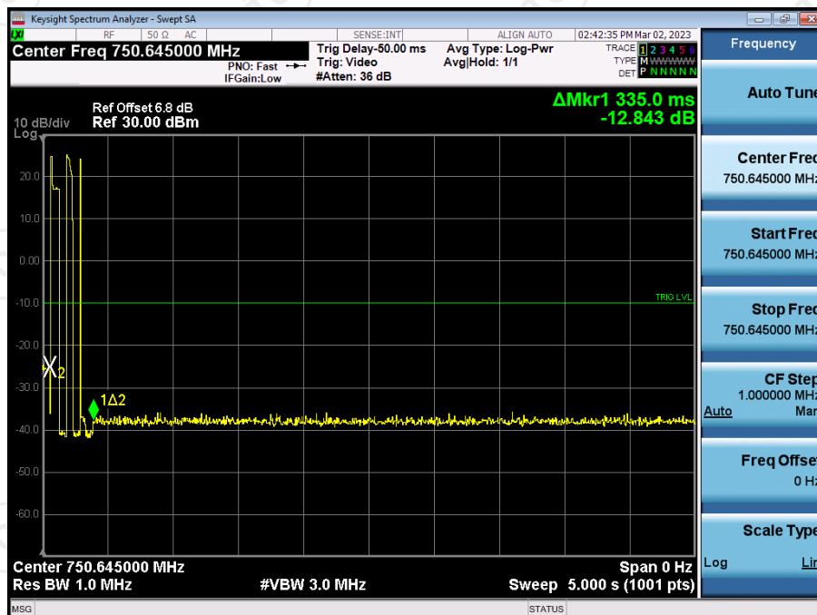
Upper700MHz DL
