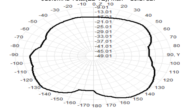
910.0MHz Total(E2-YZ), Max= -10.17dBi
