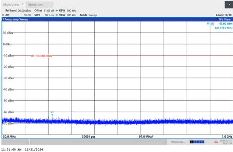
BLE_2M-Ant1-2478-30~1000-PASS
