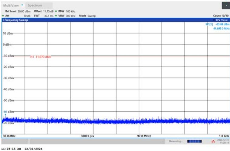
BLE_2M-Ant1-2404-30~1000-PASS
