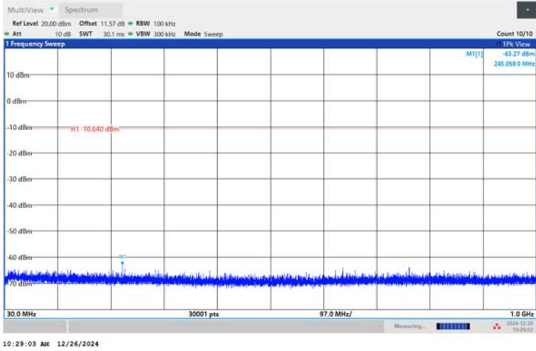
BLE_2M-Ant1-2440-30~1000-PASS
