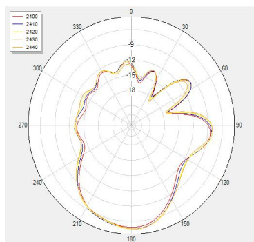
H Theta=90
