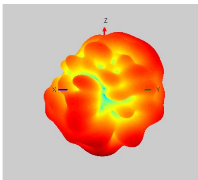
H Theta=90
