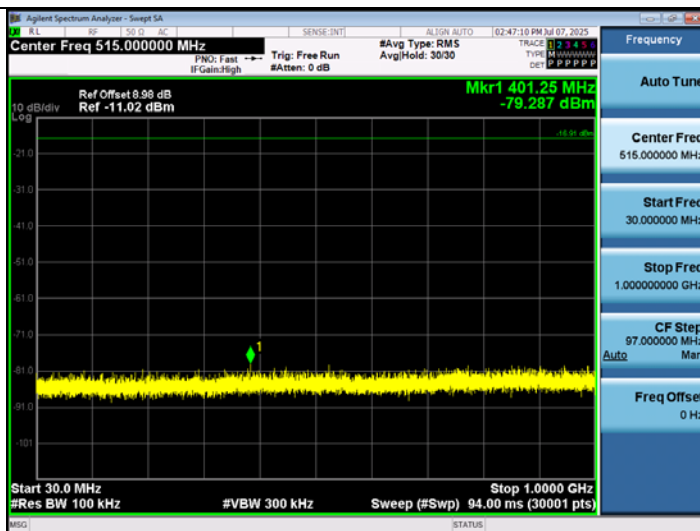
BLE 1M-Ant1-2402-30~1000-PASS
