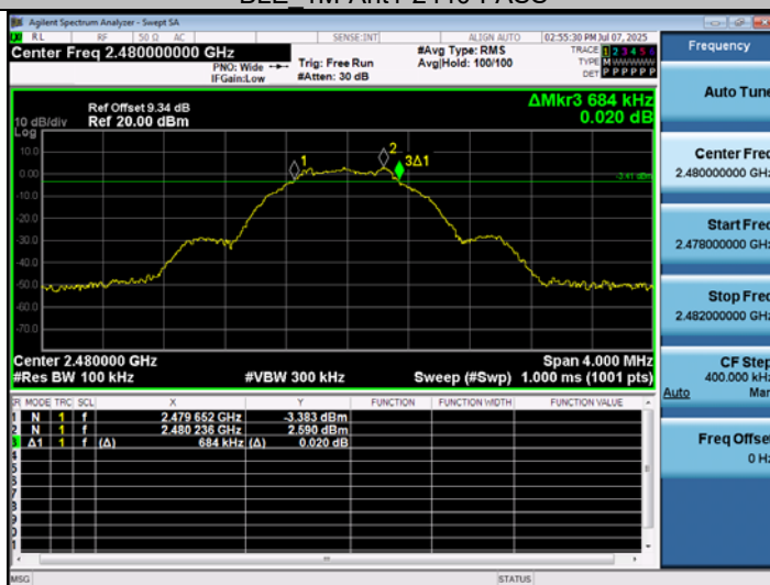
BLE 1M-Ant1-2480-PASS
