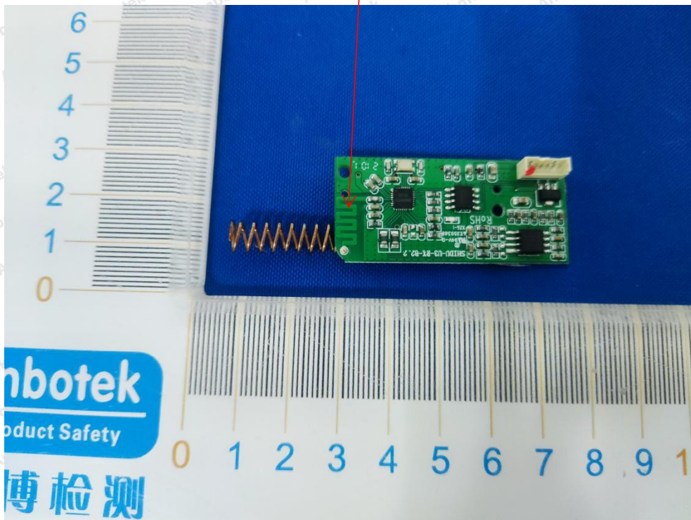
UHF ANT
