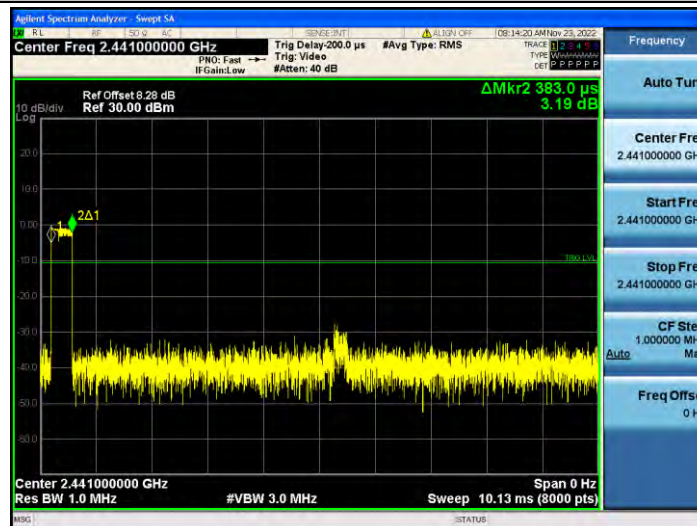
2DH1_Ant1_Hop
