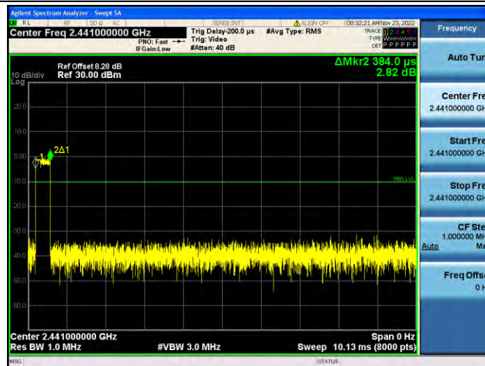
3DH1_Ant1_Hop
