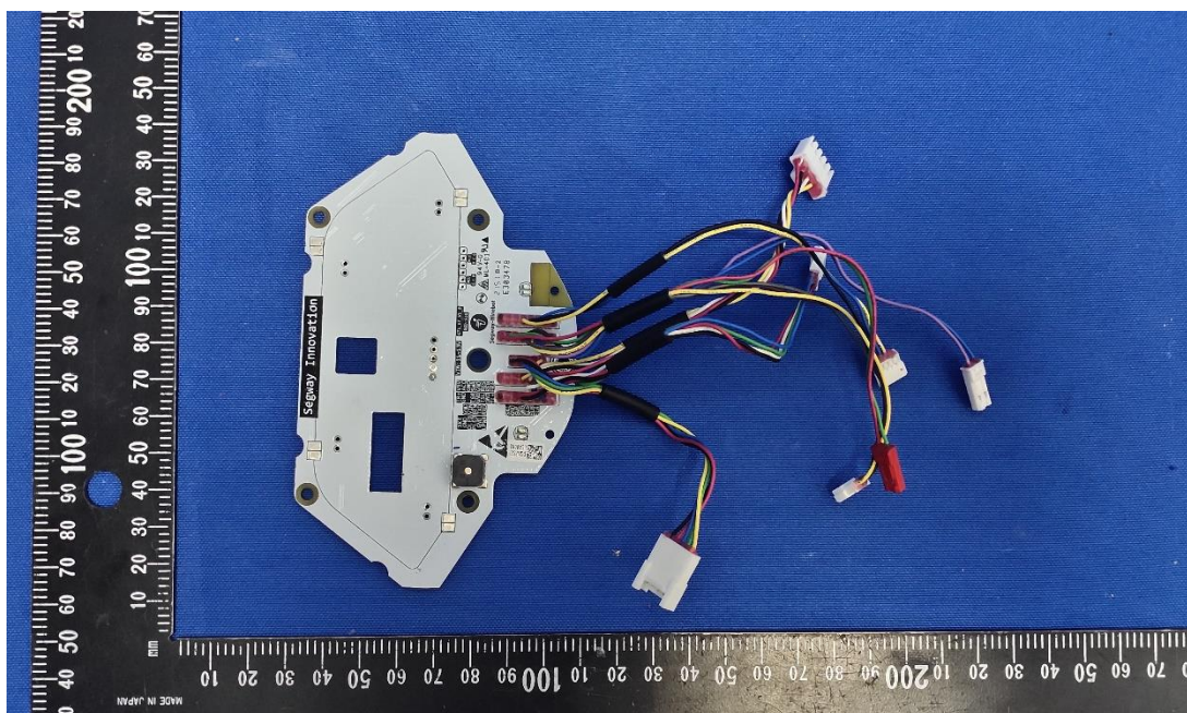
(6) EUT Photo
