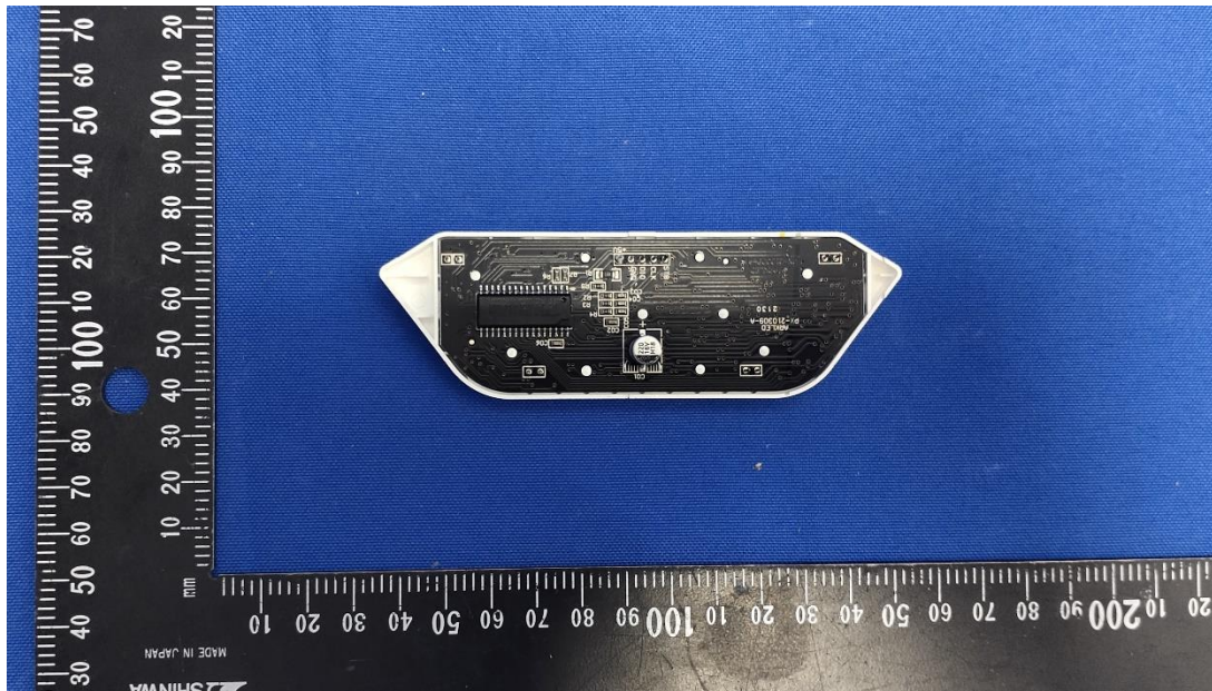
(5) EUT Photo
