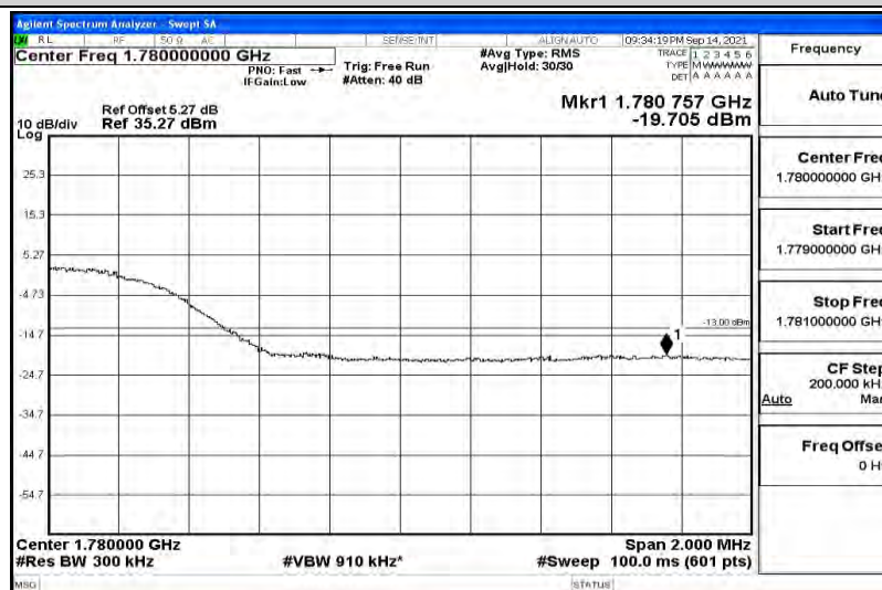
Band66-20MHz-QPSK-132072
