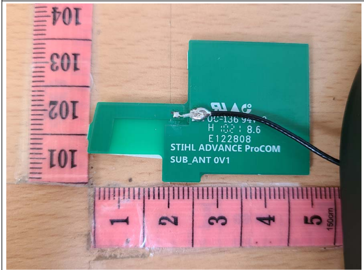
Mesh Antenna2
