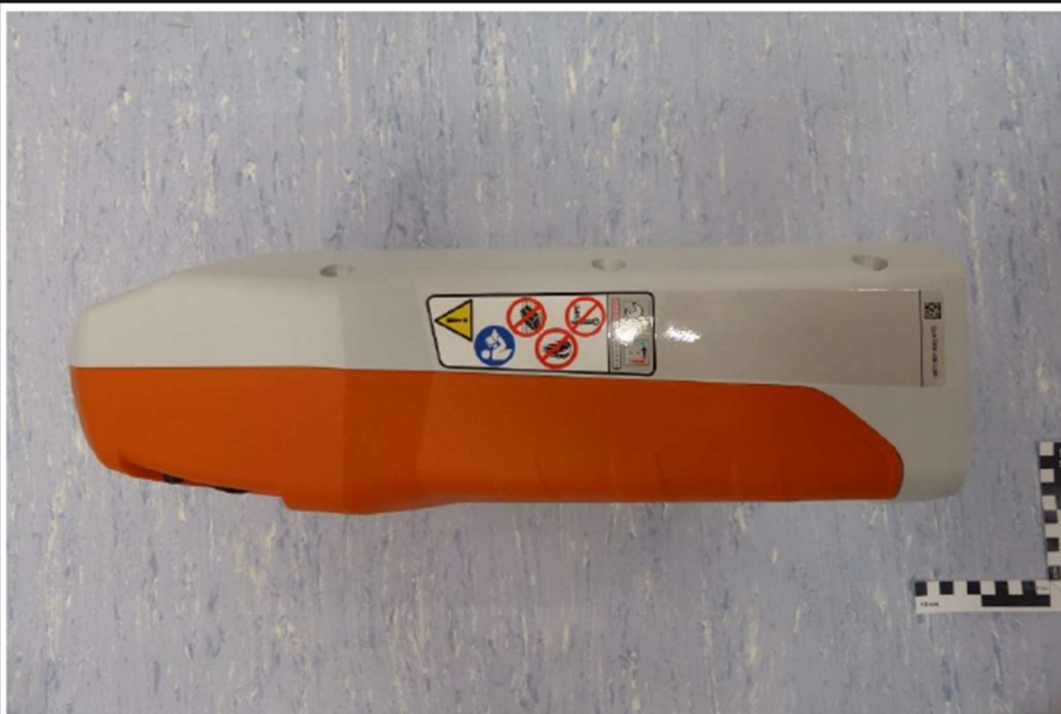
EUT RIGHT
