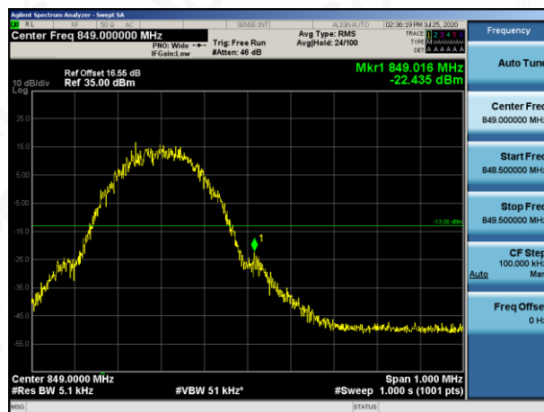
GSM 850-HCH-EGPRS
