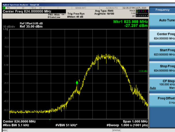
GSM 850-LCH-EPRS
