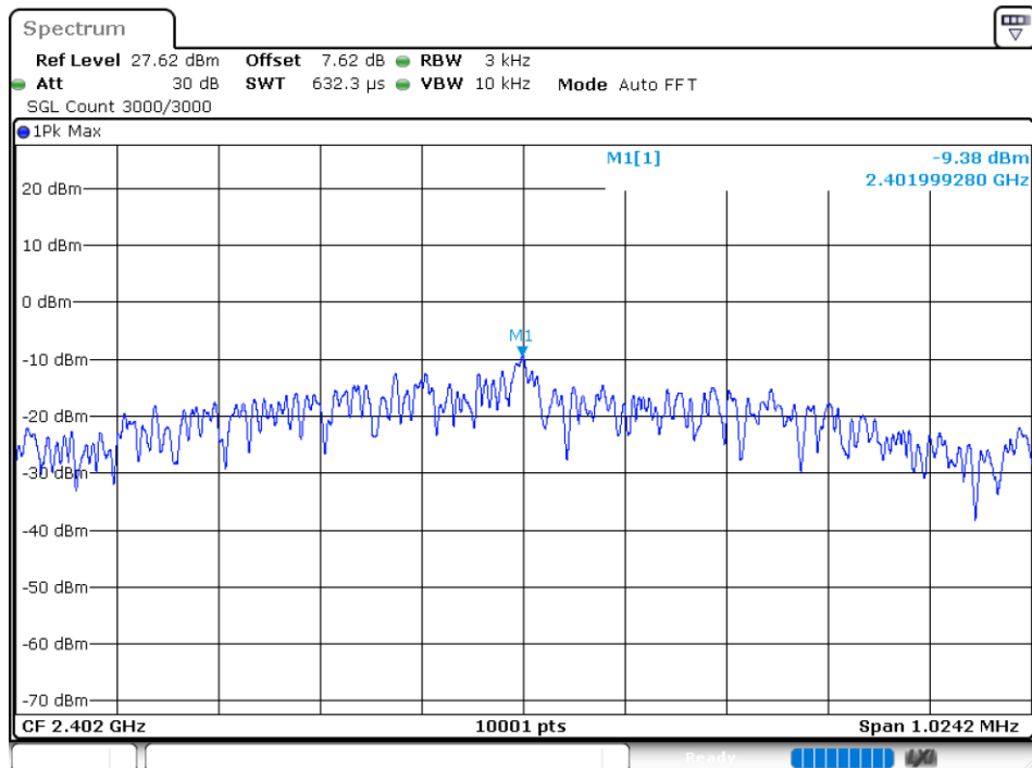
PSD NVNT BLE 2402MHz 1M
