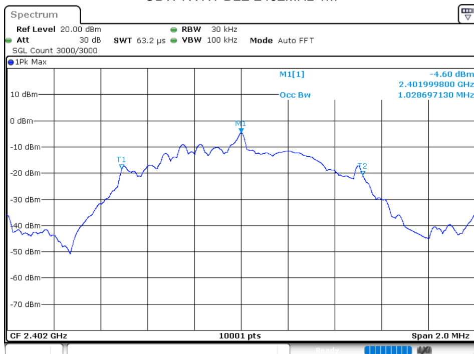
OBW NVNT BLE 2402MHz 1M
