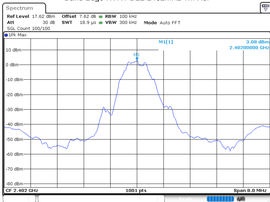
Band Edge NVNT BLE 2402MHz 1M Ref
