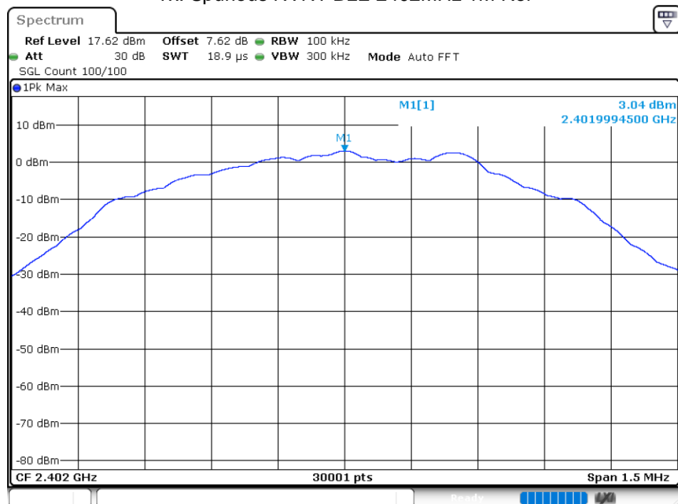
Tx. Spurious NVNT BLE 2402MHz 1M Ref
