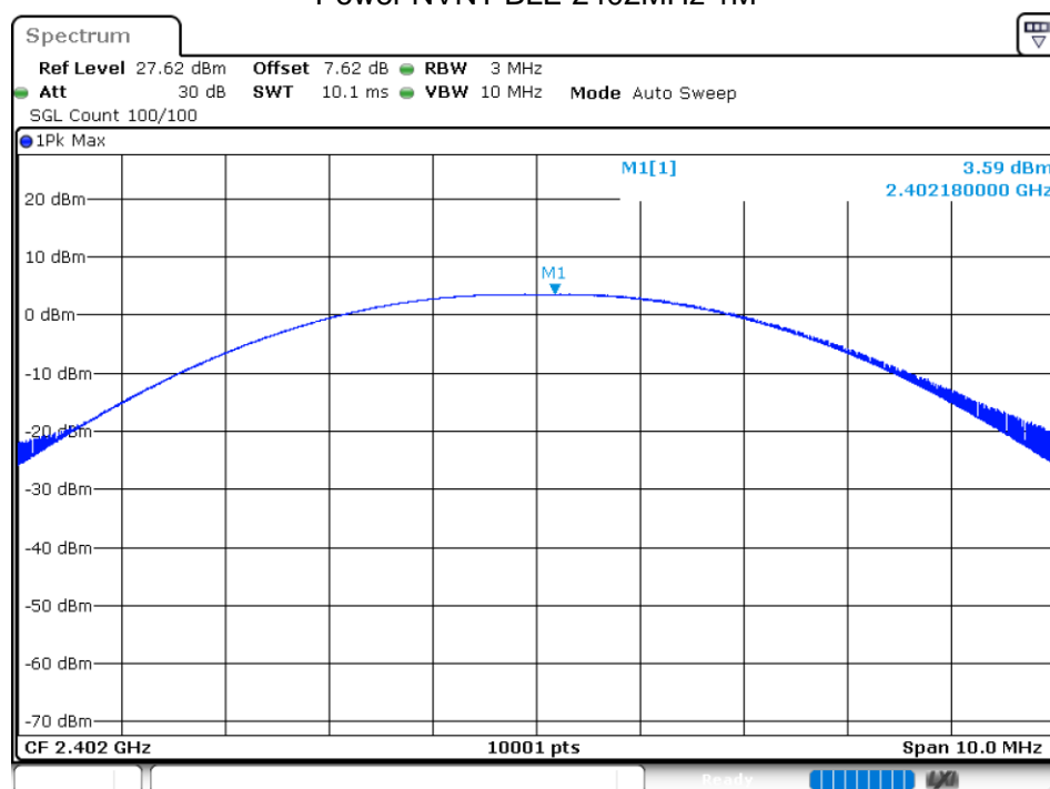
Power NVNT BLE 2402MHz 1M
