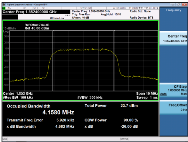
WCDMA 1900-LCH
