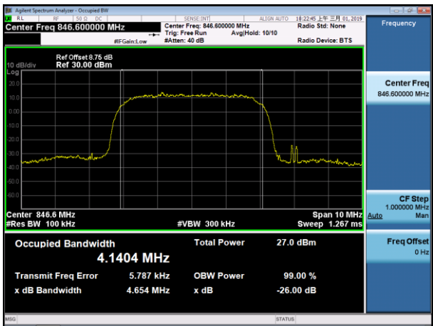
WCDMA 850-HCH
