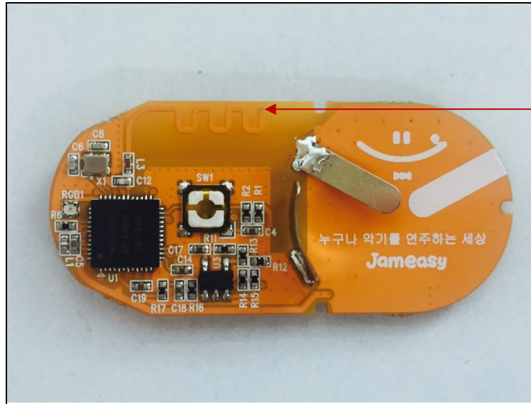
Antenna
