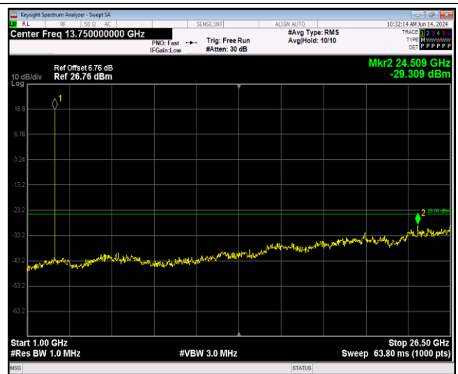
Band41-20MHz-QPSK-39750-1RB#0-Range2:1000~265 00MHz
