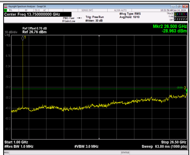
Band41-5MHz-16QAM-41565-1RB#0-Range2:1000~265 00MHz
