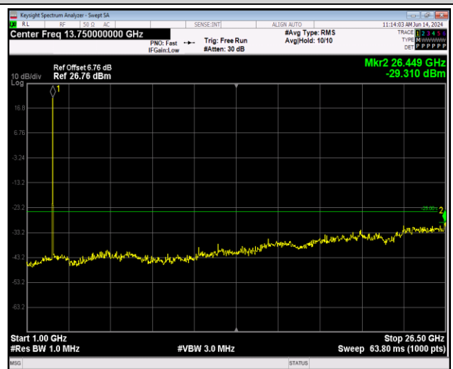
Band41-20MHz-QPSK-40620-1RB#0-Range2:1000~265 00MHz
