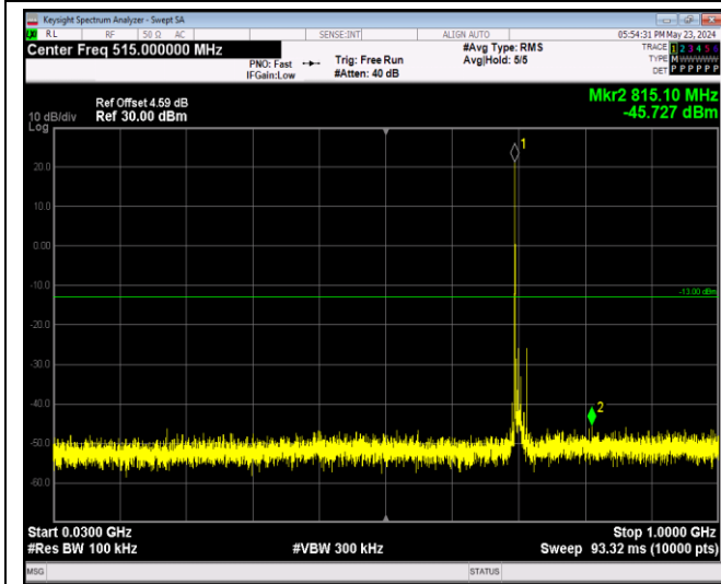
Band12-10MHz-QPSK-23095-1RB#0-Range1:30~100 0MHz
