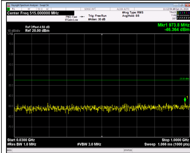
Band41-20MHz-QPSK-40620-1RB#0-Range1:30~100 0MHz
