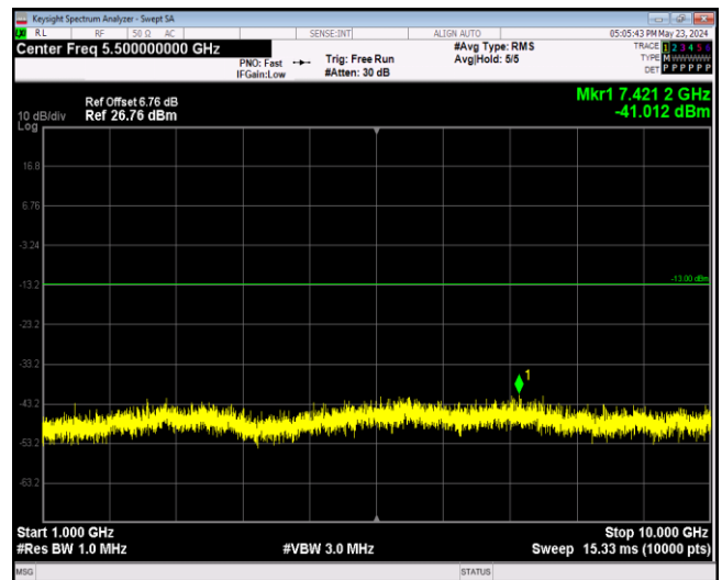
Band12-1.4MHz-16QAM-23017-1RB#0-Range2:1000~10 00MHz
