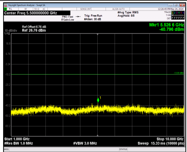
Band13-5MHz-QPSK-23255-1RB#0-Range2:1000~1000 OMHz
