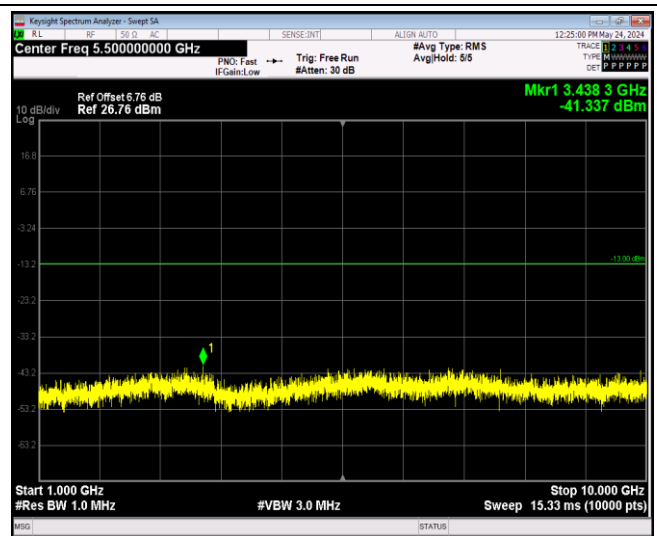
Band13-5MHz-QPSK-23230-1RB#0-Range2:1000~1000 OMHz
