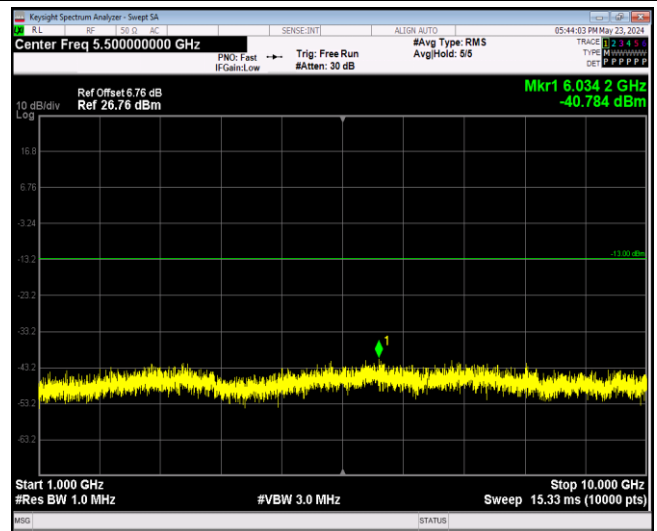
Band12-10MHz-QPSK-23095-1RB#0-Range2:1000~100 00MHz
