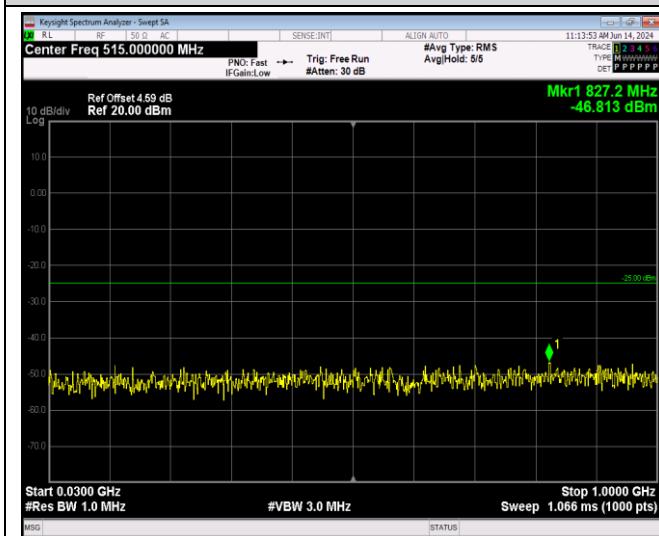
Band41-20MHz-QPSK-40620-1RB#0-Range1:30~100 0MHz
