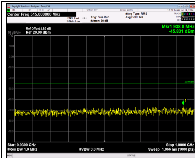
Band41-20MHz-QPSK-39750-1RB#0-Range1:30~100 0MHz
