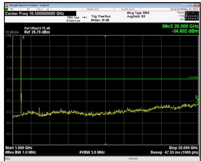
Band2-20MHz-64QAM-19100-1RB#0-Range2:1000~200 00MHz
