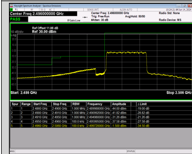
Band41-5MHz-64QAM-41565-1RB#24
