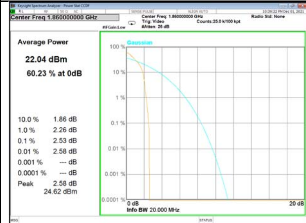
Band 2_1_Q16_Low
