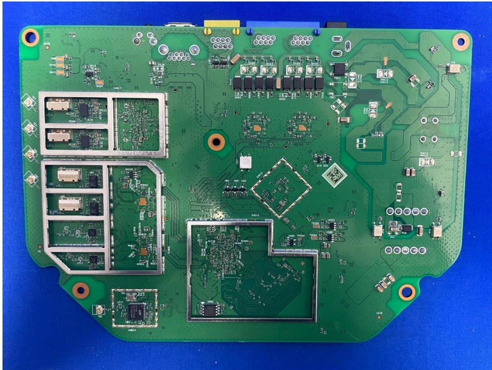
(21) EUT Photo (AP411)
