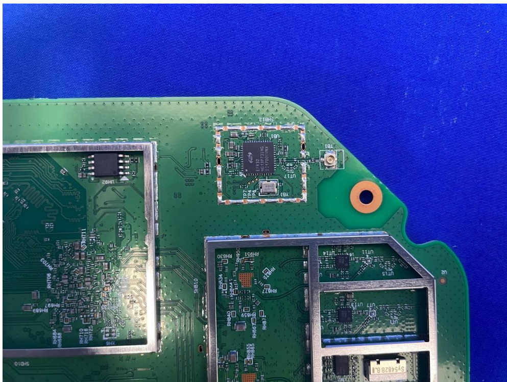
(22) EUT Photo (AP411)
