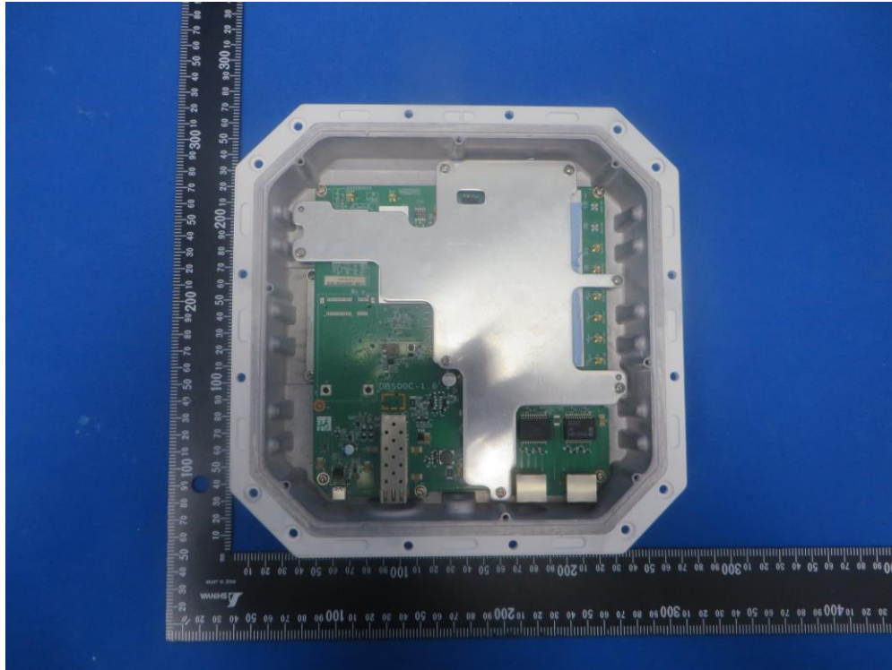
(3) EUT Photo - AP361
