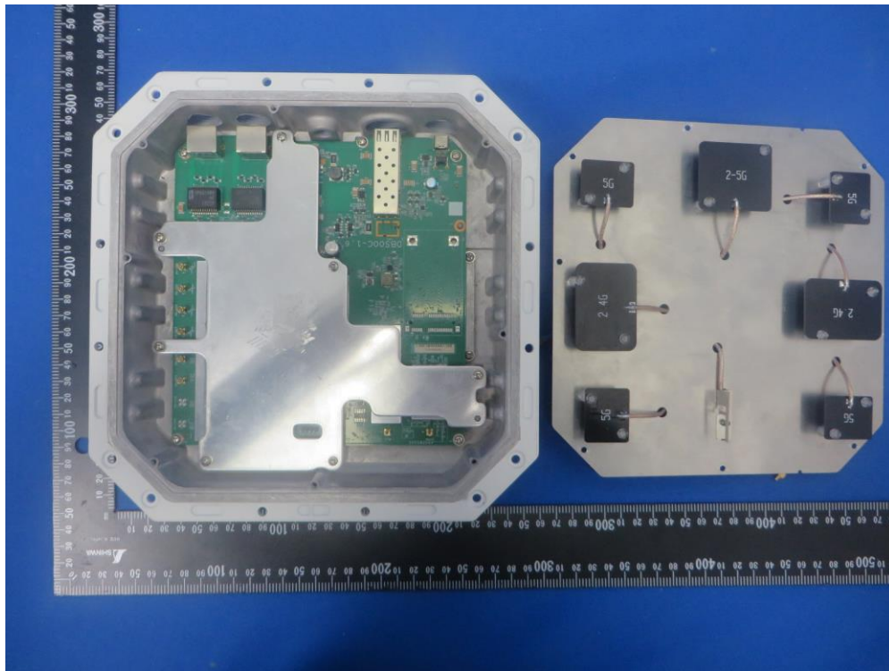
(5) EUT Photo - AP361D
