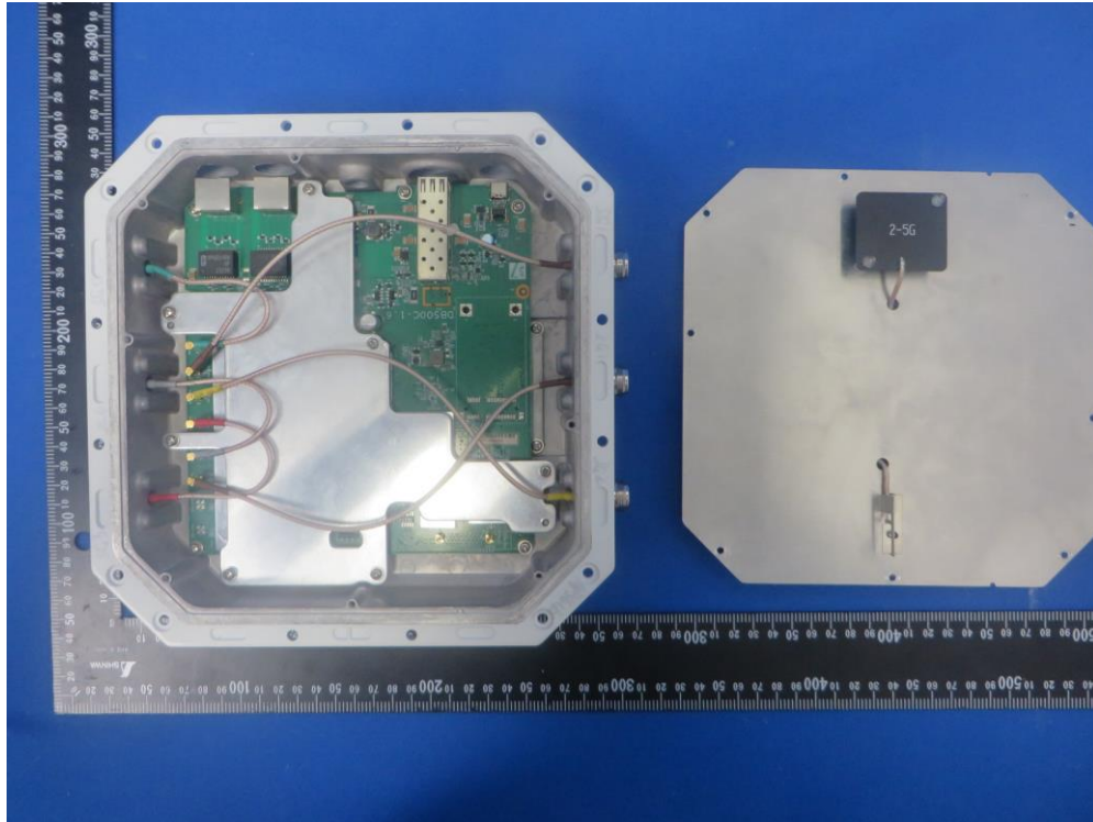
(7) EUT Photo - AP361e
