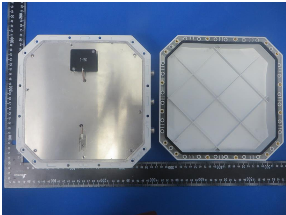
(6) EUT Photo - AP361e
