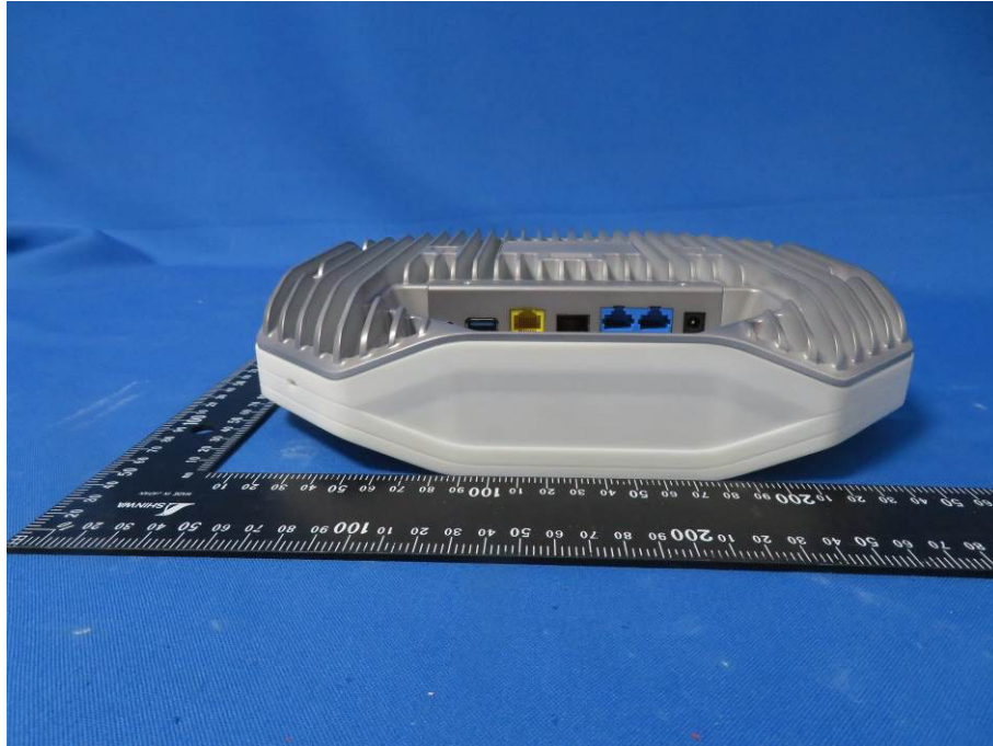
(3) EUT Photo
