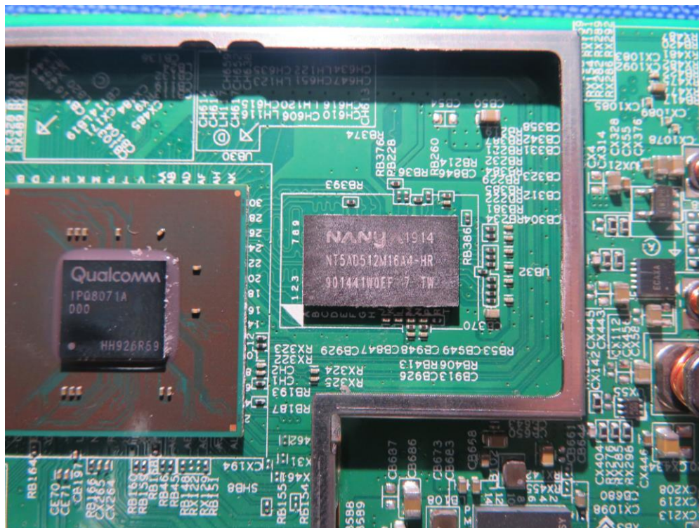
(12) EUT Photo_AP321e
