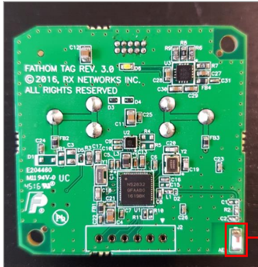
PCB Bottom
