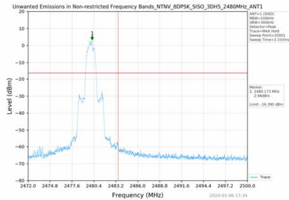
8DPSK_2480MHz_3DH5_SISO_ANT1
