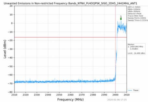
Pi/4DQPSK_Hopping_2DH5_SISO_ANT1
