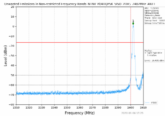
Pi/4DQPSK_2402MHz_2DH5_SISO_ANT1
