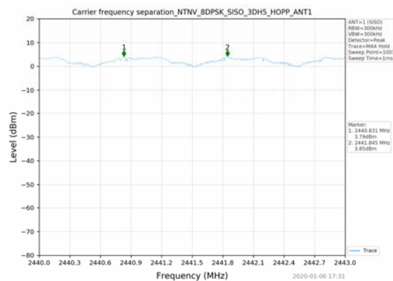
8DPSK_Hopping_3DH5_SISO_ANT1
