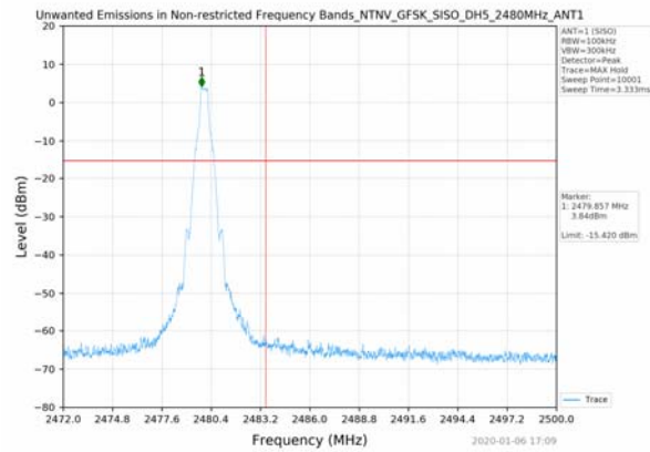
GFSK_2480MHz_DH5_SISO_ANT1
