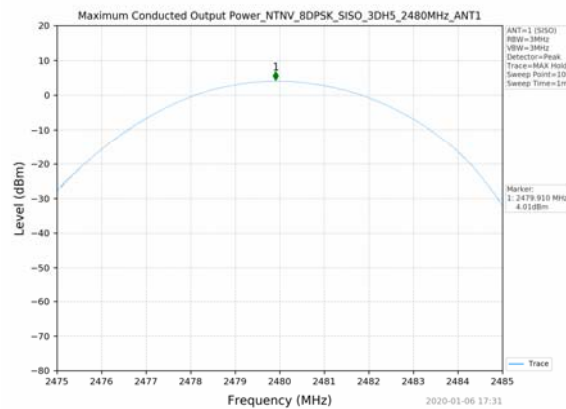
8DPSK_2480MHz_3DH5_SISO_ANT1
