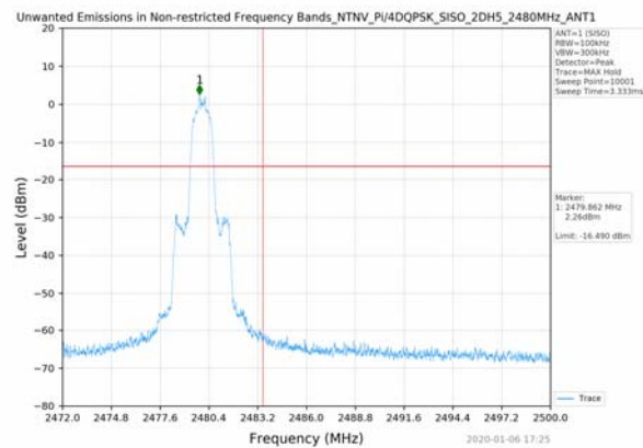
Pi/4DQPSK_2480MHz_2DH5_SISO_ANT1
