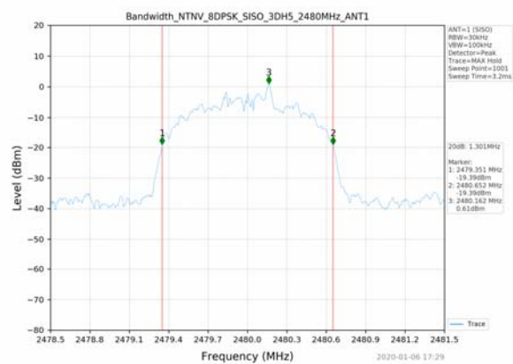
8DPSK_2480MHz_3DH5_SISO_ANT1
