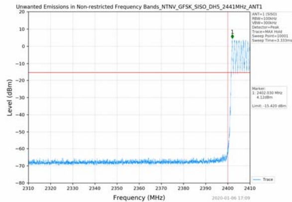
GFSK_Hopping_DH5_SISO_ANT1
