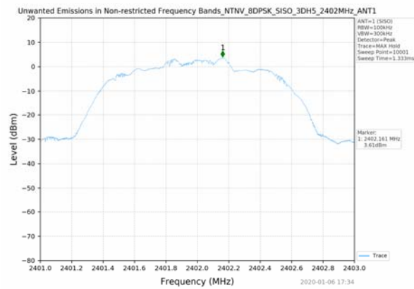
8DPSK_2402MHz_3DH5_SISO_ANT1
