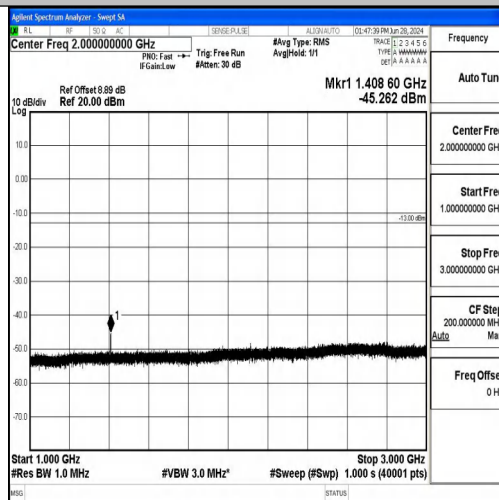
Band17 5MHz QPSK 23755 1RB#0 1000~3000 1000~3000
