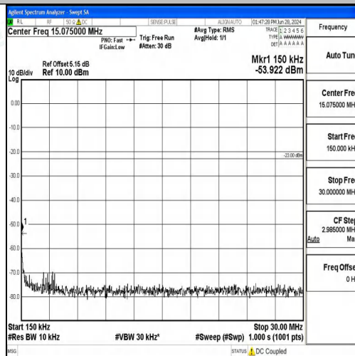
Band17 5MHz QPSK 23755 1RB#0 0.15~30 0.15~30
