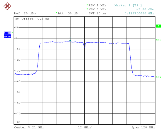
802.11ac(HT80) Low channel
