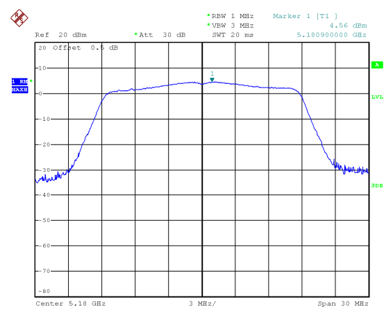
802.11ac(HT20) low channel
