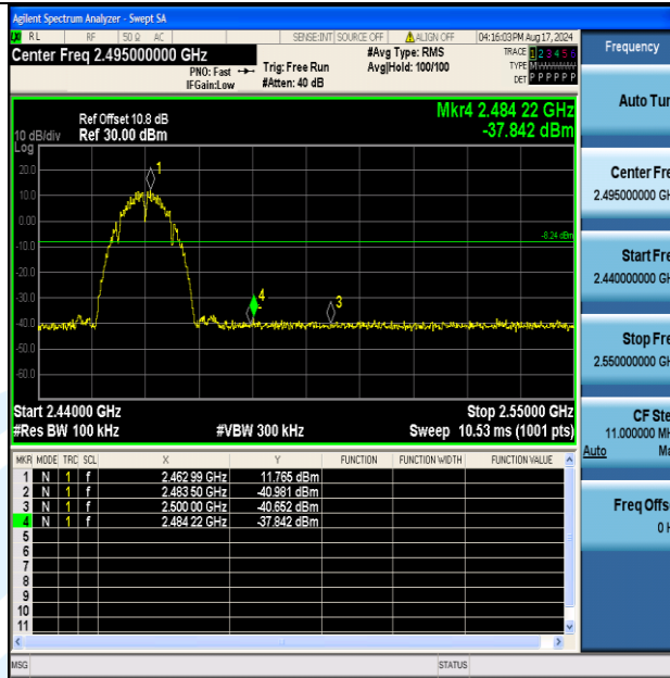
11B-Ant2-2462-PASS
